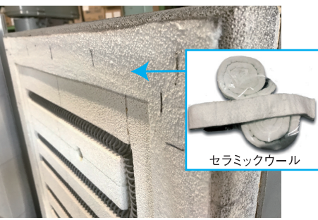
扉パッキン
